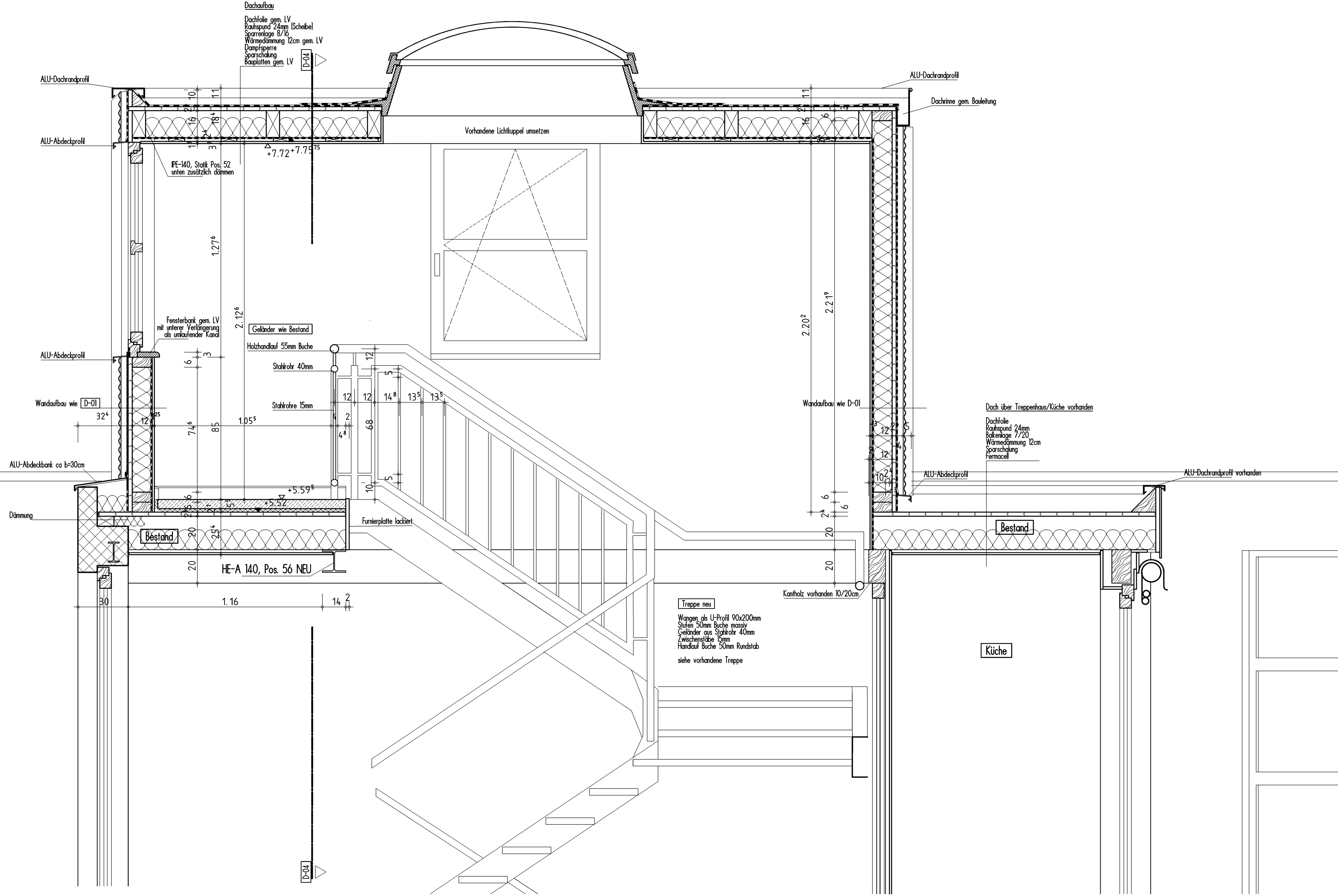
D-05 Querschnitt Treppenhaus 2.OG M1:10
