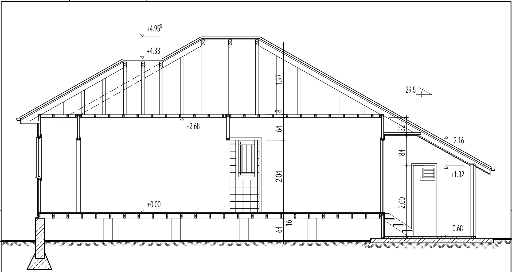
A-A Cut - M 1:50
