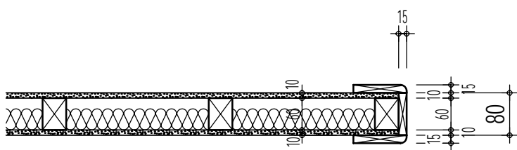
Door Inner Wall - M 1:10
